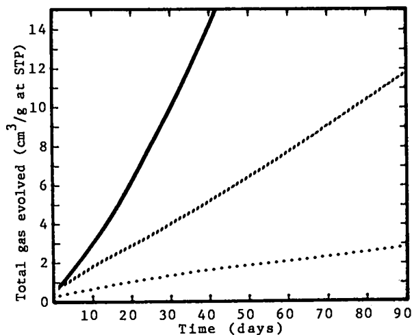
Fig. 7. DPBT (Dipicrylbenzobistriazolidione)
