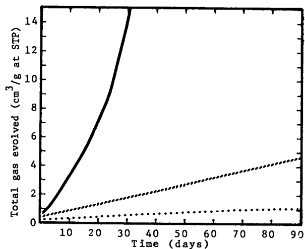
Fig. 1. ABH (Azobishexanitrobiphenyl)
