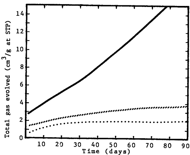
Fig. 4. DATB (Diaminotrinitrobenzene)
