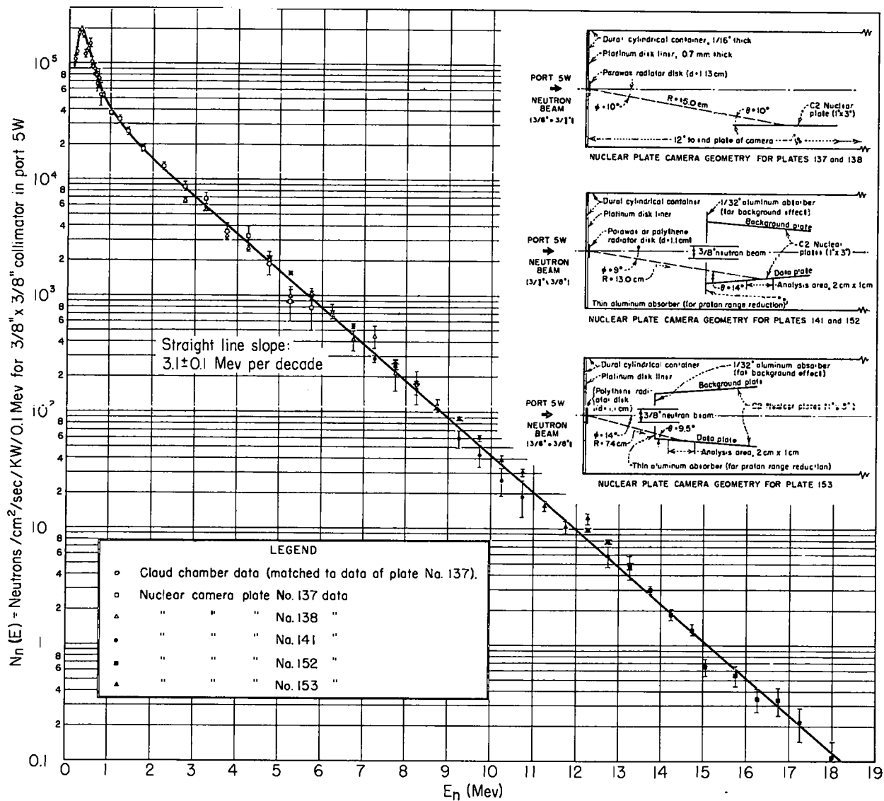
Fig. 56. Fast neutron spectrum.
