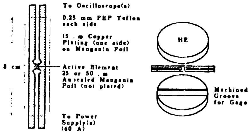
Fig. 2. Manganin gauge.
